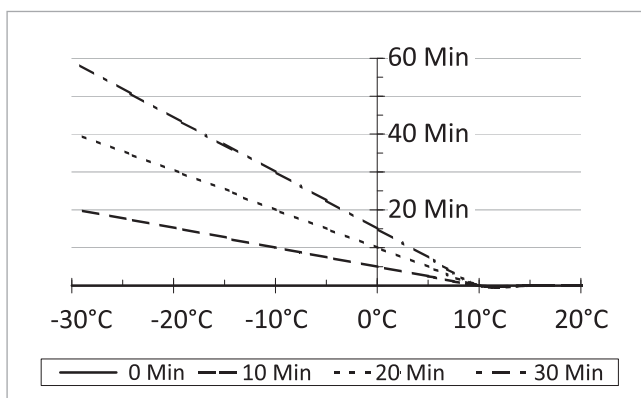
Abb. 8: Vorhaltezeit
