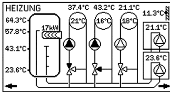
Abb. 10: Beispiel SolvisMax (SolvisBen anderes Schema)
