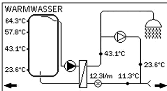
Abb. 9: Beispiel SolvisMax (SolvisBen anderes Schema)
