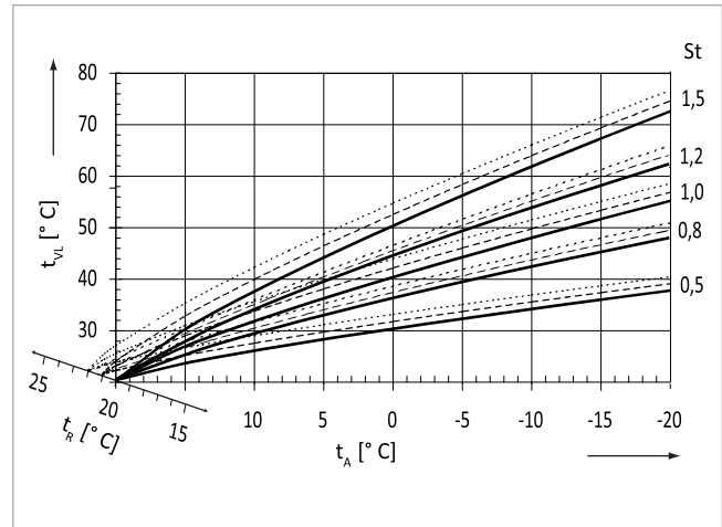
Abb. 7: Heizkurven bei diversen Raumsolltemperaturen
