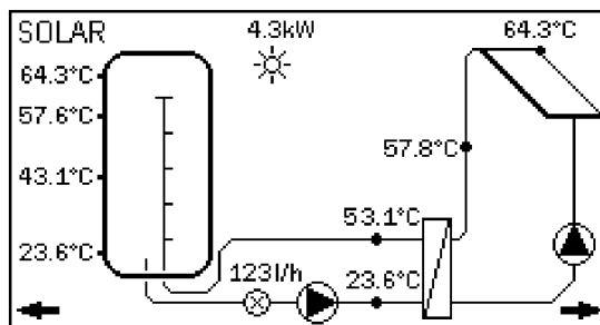
Abb. 11: Beispiel SolvisMax (SolvisBen anderes Schema)
